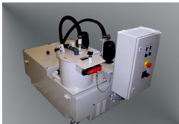
installation compacte avec MR 25 pour petites machines-outils
