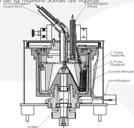
principe de fonctionnement de la MR 25
