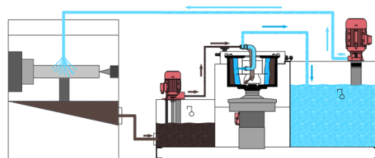
带磁吸预处理的T22过滤系统
